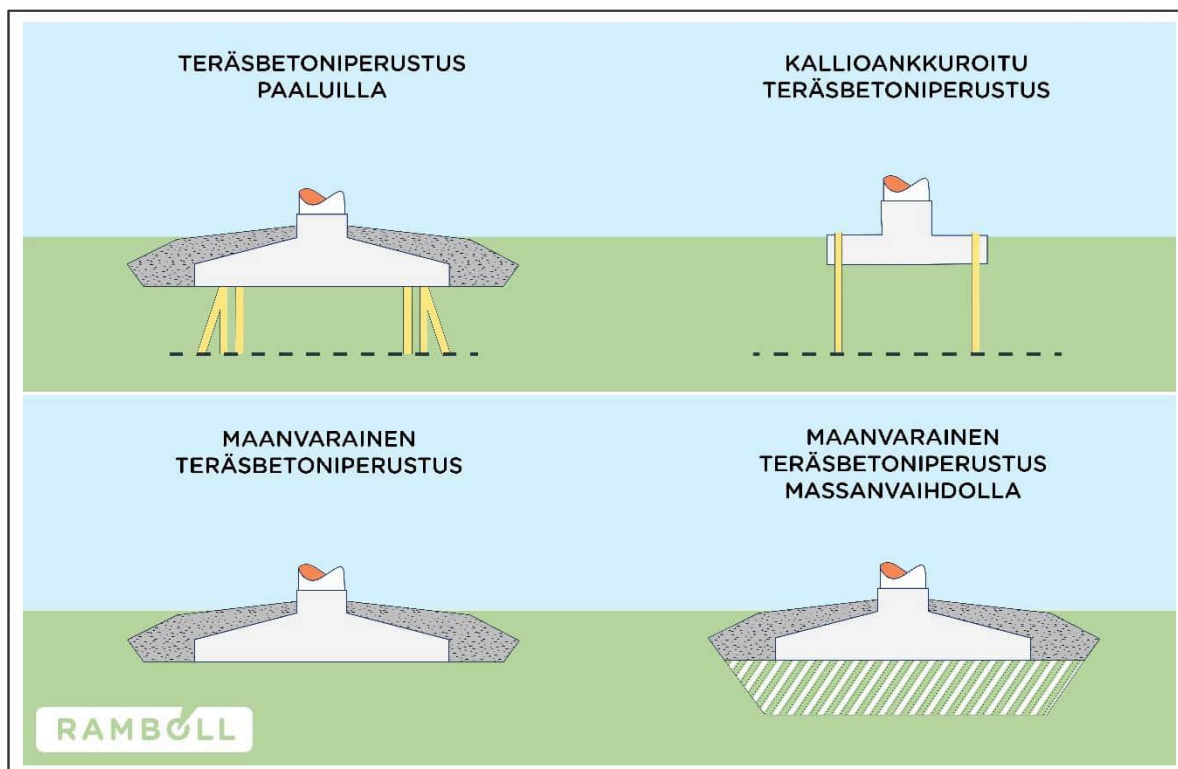
Kuva 6-2. Tuulivoimaloiden perustamistekniikoita.
