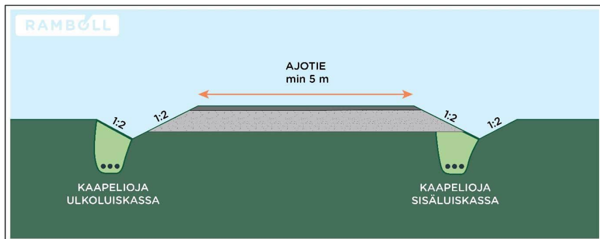
Kuva 6-4. Ajoteiden ja kaapeliojien periaatekuva.
