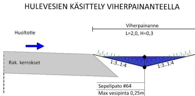
Kuva 6 Esimerkki ojakatkoista (Virginia Stormwater Management Program) ja tyyppileikkaus huoltoteiden yhteyteen rakennettavista viherpainanteista
