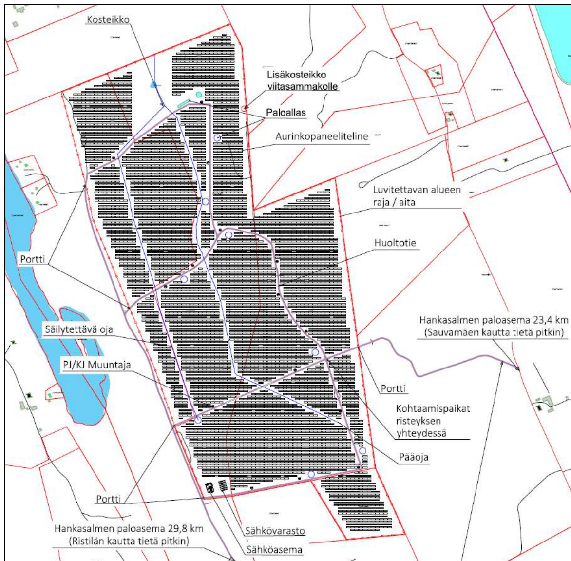
Kuva 2. Asemapiirros, jossa paloaltaat, tiet, portit, paneelialueet ja Pien-/keskijännite muuntajat ym.
