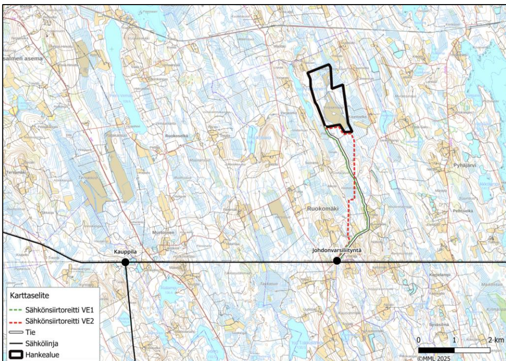
Kuva 13. Viroensuu sähkösiirtoreitit maakaapelein (2 kpl, WestWind, Liite 8.3)
