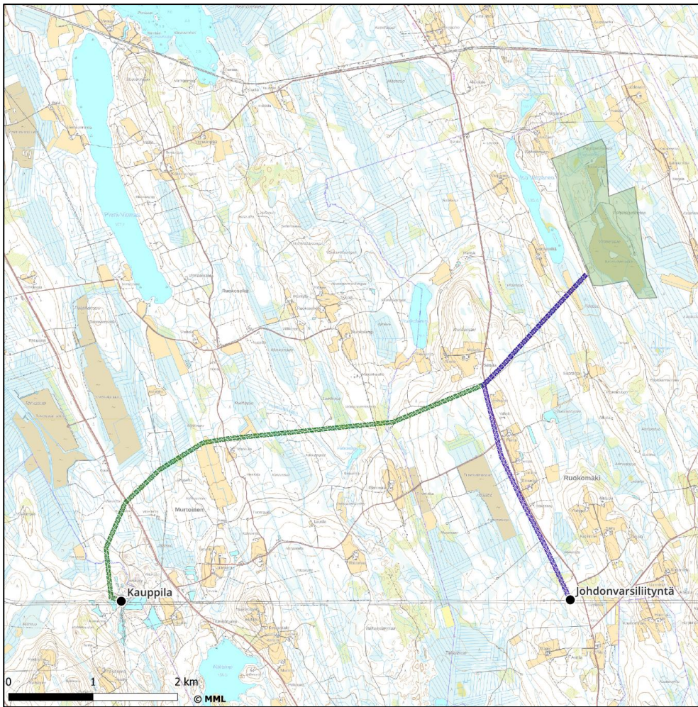
Kuva 12. Viroensuu sähkösiirtoreitit (2 kp, Sitema Oy, I ks. Liite 8.1 ja 8.2)
