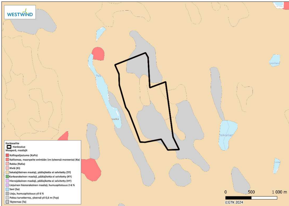
Kuva 25. Geologian tutkimuskeskuksen maaperäaineisto (1:200 000).
